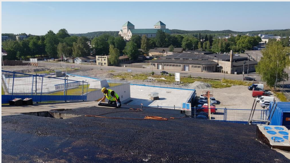
C-talon katon höyrynsulkukermin asennusta. Tätä ennen betonipintaan on sivelty pölynsidontaa varten pikimassaa. (kuva 26.7.18)
