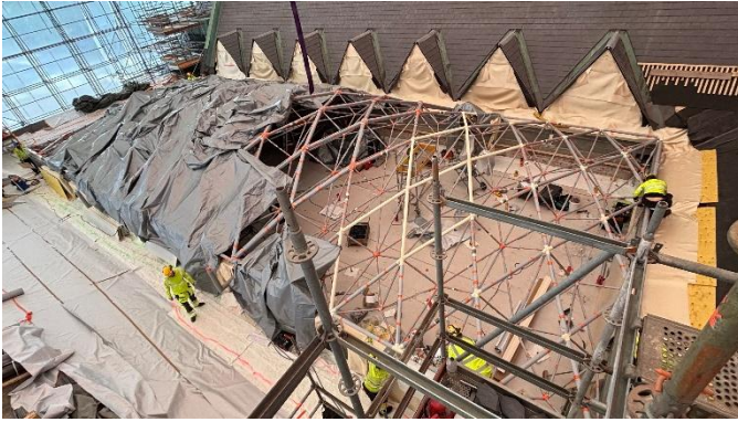
Kuva 5. Halkopihan lasikaton metallikehikko nostettu paikoilleen ja hitsaustyöt käynnissä pressun alla.
