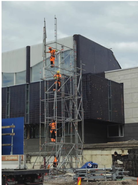
Kuva 2. Sääsuojatelineiden purkua
