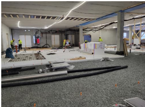
Kuva B -lohkon lattian eristys ja rauditus
