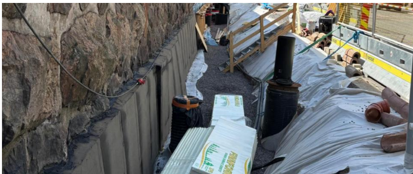
Kuva 8. Vaunuvajan sokkelitöitä.
