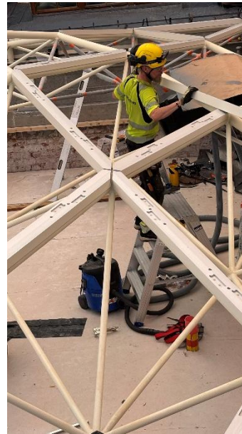
Kuva 9. Halkopihan lasikaton alumiiniprofiilien asennusta.
