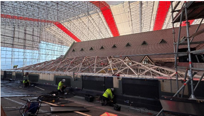
Kuva 8. Halkopihan lasikatoksen sokkelin pellitystä.
